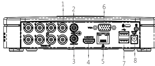
DHI-XVR5108C-S2
